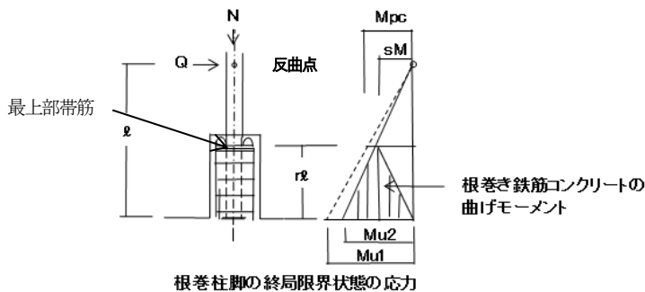
根巻柱脚の終局限界状態の応力
