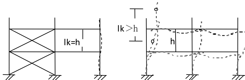
① 水平移動拘束されているラーメン
